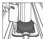
5. Fijar DEKTITE® con tornillos autotaladrantes EJOT® o remaches Bulbtite.
