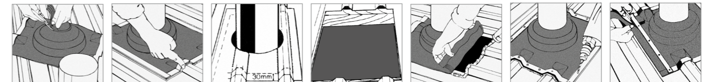
1. Ajuste Dektite® al tubo. 2. Ajuste Dektite® a la chapa perfilada y marque. 3. Marque la línea exterior del Dektite® Soaker en la cubierta. Retire el Dektite® y marque una franja extra de 30 mm. 4. Corte y retire la cubierta dentro del área marcada a 30 mm. Lime los bordes afilados. Pueden instalarse soportes de madera para sujetar el tejado donde los refuerzos de la chapa se han eliminado. 5. Aplique sellante y ajuste el Dektite® con precisión a la chapa perfilada. 6. Fijar primero en las cimas empezando los centros de los lados. Siga hacia los extremos. 7. Use las tiras metálicas de perfil suministradas para sellar los bordes solapados. Corte hacia los cuatro lados sobrantes.
