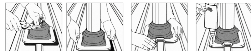
1. Ajuste Dektite® al tubo. 2. Ajuste Dektite® a la chapa perfilada y marque. 3. Adapte Dektite® a la forma de la chapa perfilada. 4. Fije Dektite® con tornillos autotaladrantes EJOT® o remaches Bulbrite.
