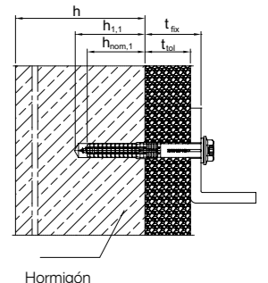
Hormigón
