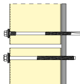
Fig. 2 Montaje de panel sándwich con fijación vista.
