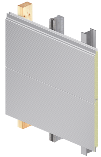
Fachada con paneles sándwich
