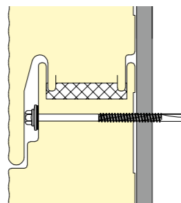
Fig. 1 Montaje de panel sándwich con fijación oculta.
