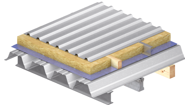
Cubierta con chapa doble perfilada
