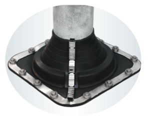
1. Ajuste Dektite® al tubo. 2. Ajuste Dektite® a la chapa perfilada y marque. 3. Marque la línea exterior del Dektite® Soaker en la cubierta. Retire el Dektite® y marque una franja extra de 30 mm. 4. Corte y retire la cubierta dentro del área marcada a 30 mm. Lime los bordes afilados. Pueden instalarse soportes de madera para sujetar el tejado donde los refuerzos de la chapa se han eliminado. 5. Aplique sellante y ajuste el Dektite® con precisión a la chapa perfilada. 6. Fijar primero en las cimas empezando los centros de los lados. Siga hacia los extremos. 7. Use las tiras metálicas de perfil suministradas para sellar los bordes solapados. Corte hacia los cuatro lados sobrantes.
