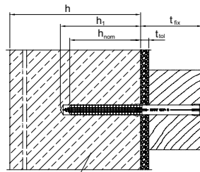
Instalación Subestructura
