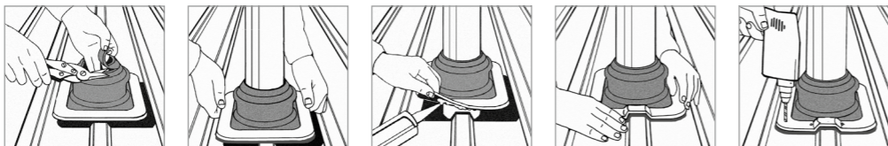
1. Ajuste Dektite® al tubo. 2. Ajuste Dektite® a la chapa perfilada y marque. 3. Aplicar compuesto sellante. 4. Adapte Dektite® a la forma de la chapa perfilada. 5. Fije Dektite® con tornillos autotaladrantes EJOT® o remaches Bulbrite.
