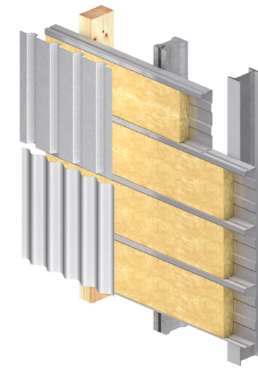
Fachada de sándwich in-situ
