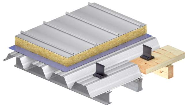
Cubierta de doble capa engatillada o clipada
