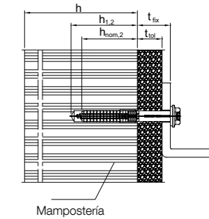
Mampostería
